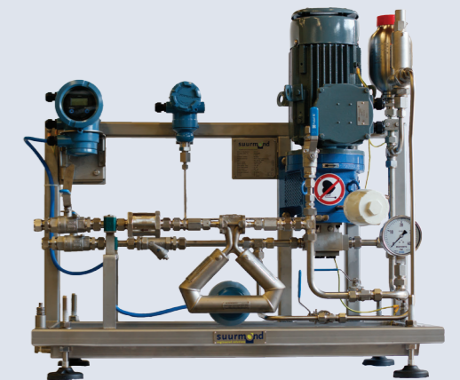
SuurDOSmini, ATEX certified
